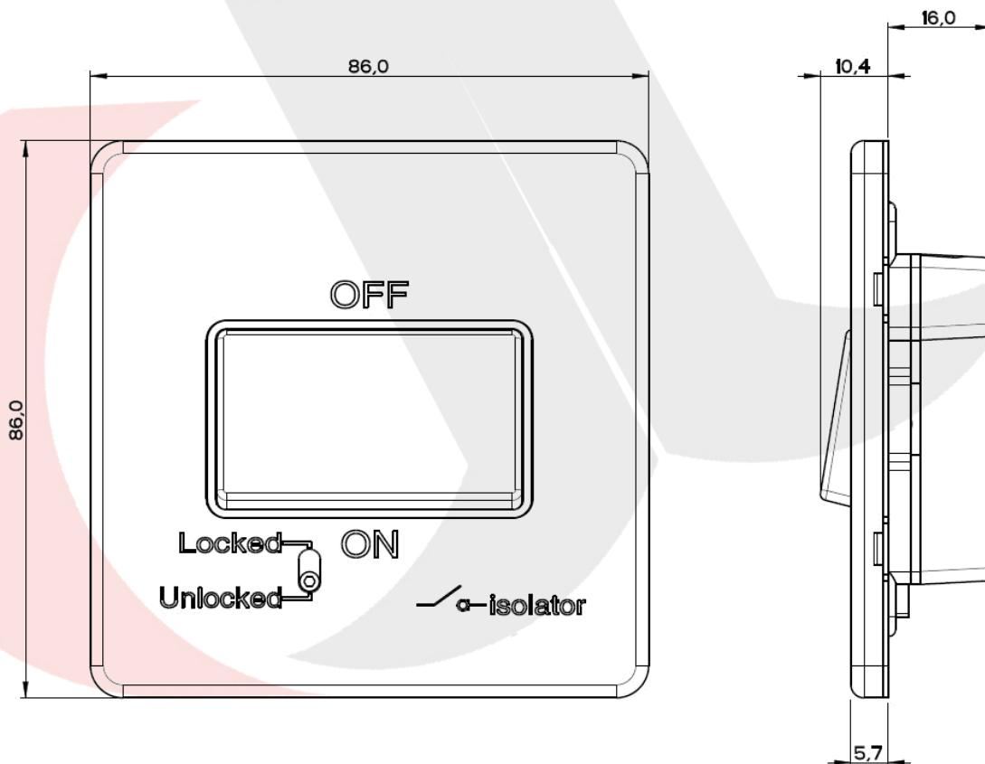
Fan Isolator Unit
